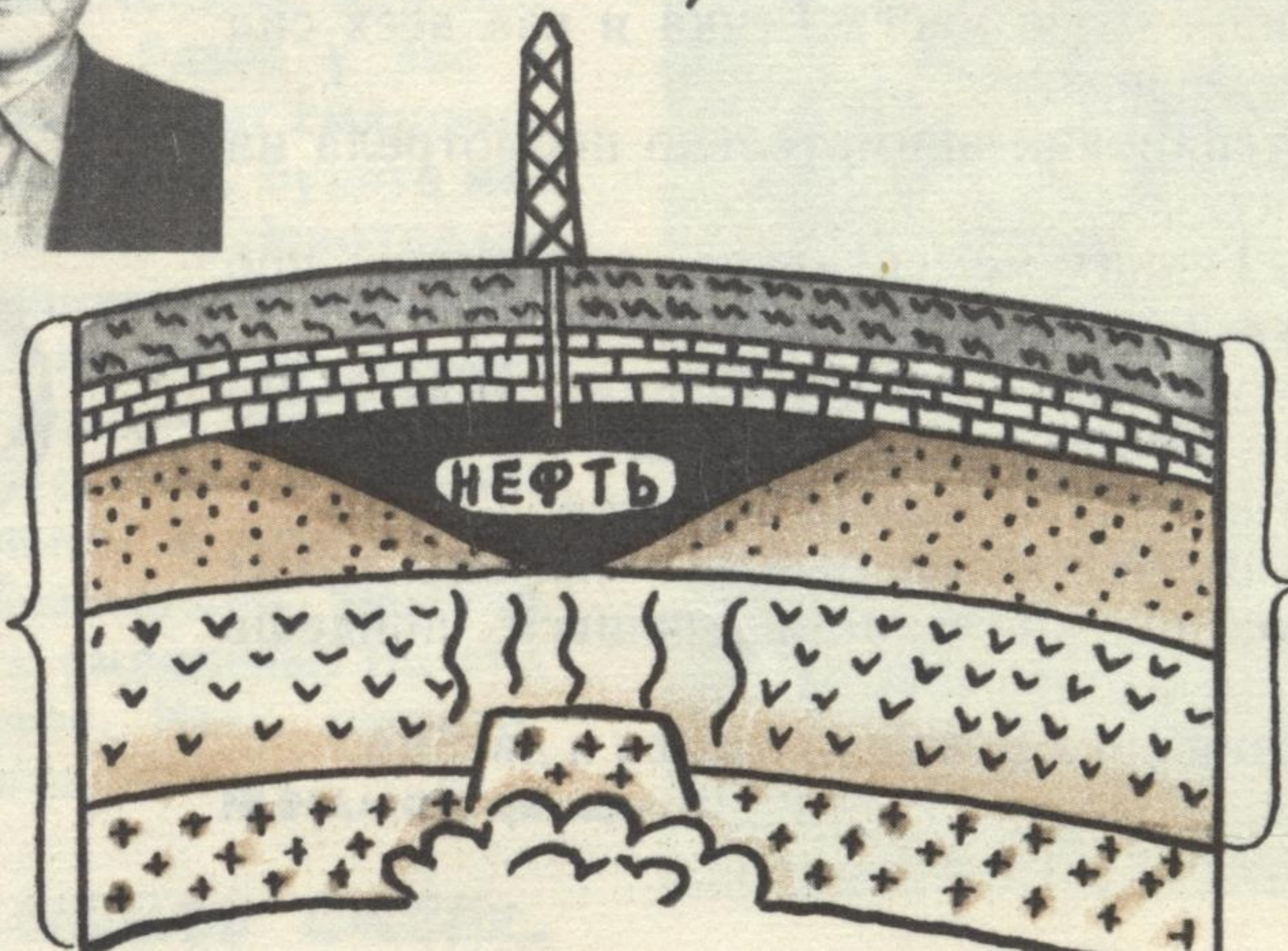
Осадочные породы
